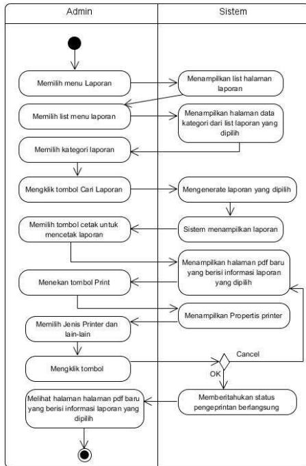
Gambar 6. Diagram Activity Membuat Laporan
