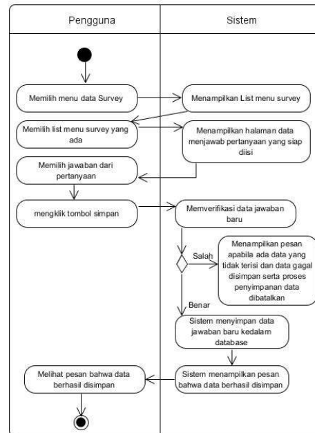
Gambar 5. Activity Diagram Menjawab Pertanyaan
