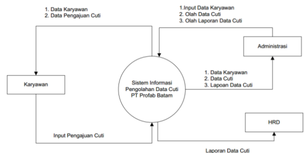
Gambar 6. Diagram Konteks
